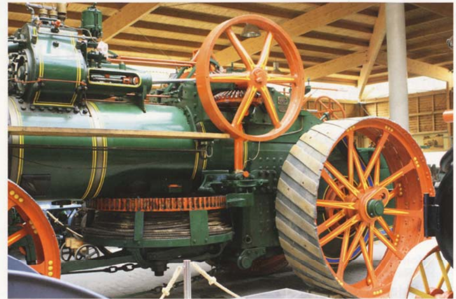
Dampfpflug-Lokomotive der Fabrik Gatersleben aus dem Jahr 1911 (Foto: G. Seyffert)
